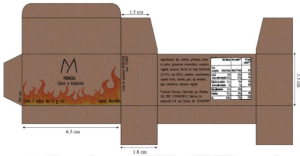
Figura 5.1 Diseño del envase
