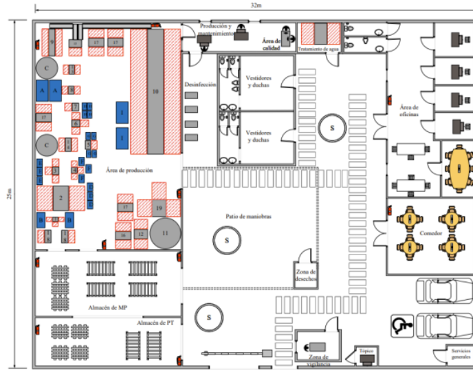
Figura 5.15 Plano de planta
