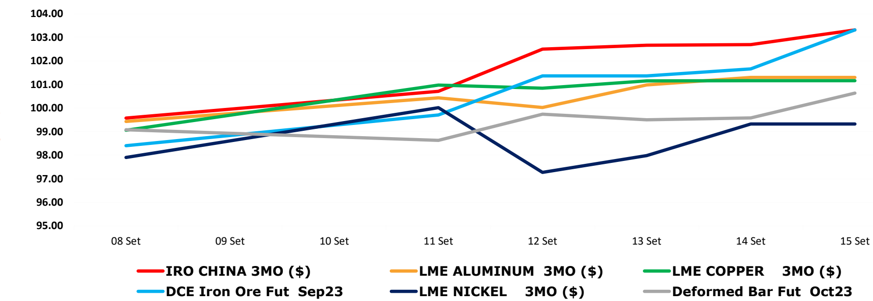
Trayectoria de los metales (7 días)
